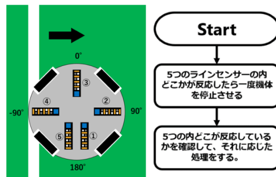
図9 ラインセンサー制御
