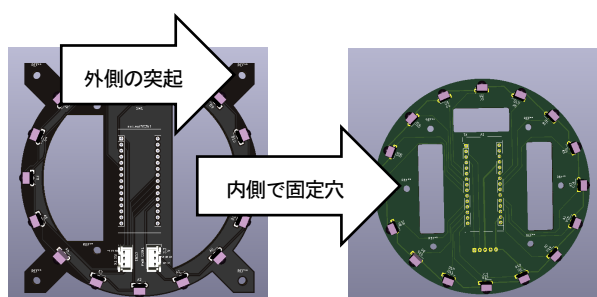
前回のIRセンサー.
